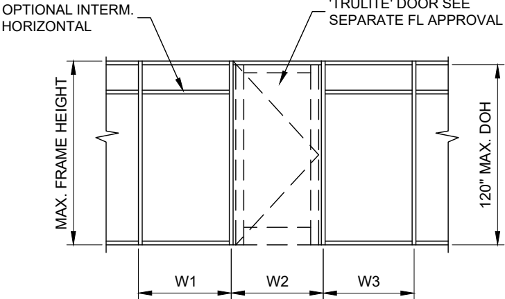
ELEVATION E4
