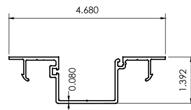
A5 OPEN BACK MULLION FILLER CG501-5
