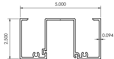
A1 JAMB / HEAD CG501-11
