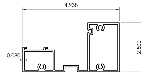
A2 SILL/HEAD CG501-2
