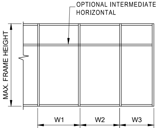
ELEVATION E1
